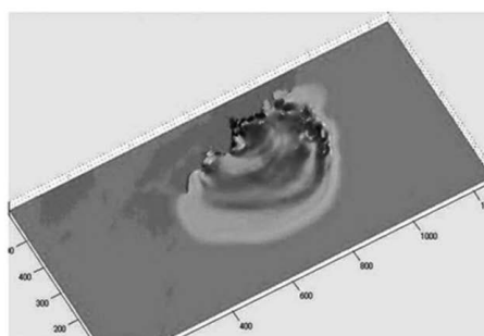
図2 東南海沖地震による津波の発生と伝播のシミュレーションの一例：日本列島周辺の津波来襲までの時間と津波高での予測を数値計算により行う。東南海地震による津波では、東海地方から西国、九州沿岸まで広い範囲での津波の被害が予想されている。
