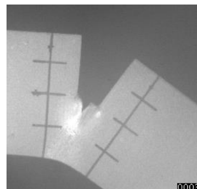
高速き裂進展現象の観察例
